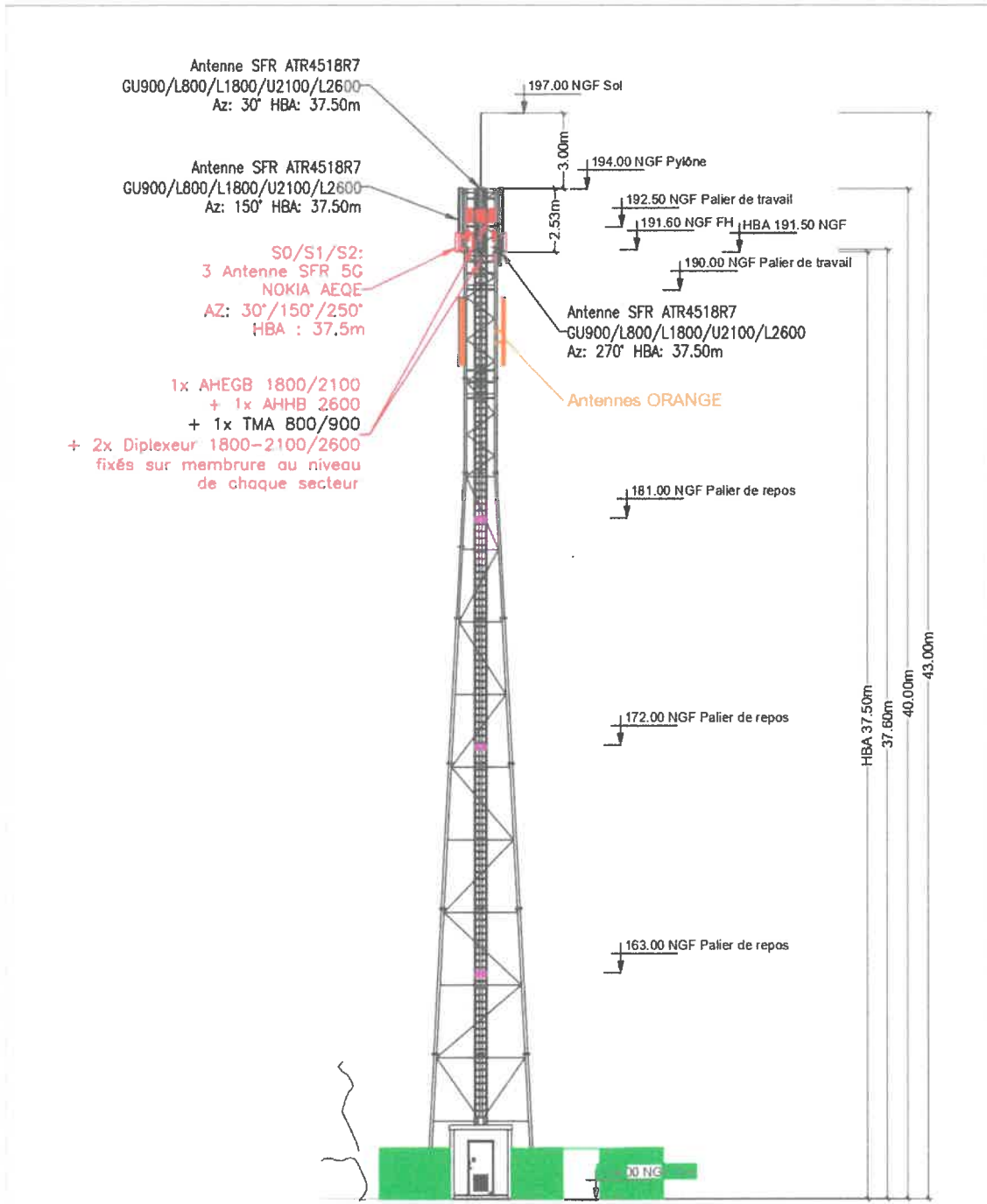
ELEVATION NORD OUEST
